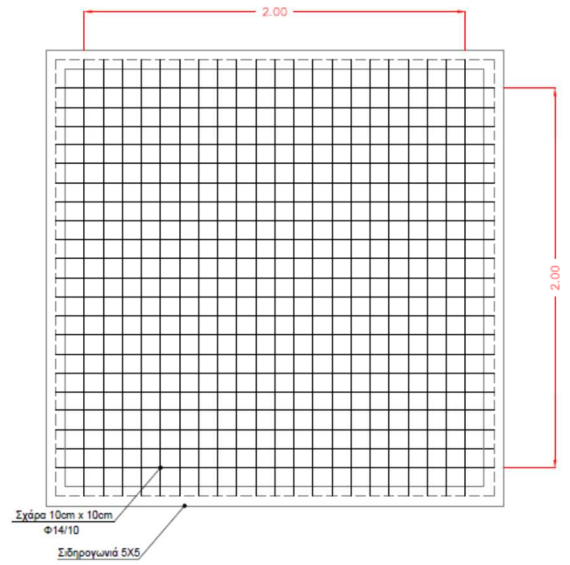
ΤΥΠΙΚΟ ΚΑΛΥΜΜΑ ΑΣΦΑΛΙΣΗΣ ΦΡΕΑΤΙΩΝ [2.0m x 2.0m]
