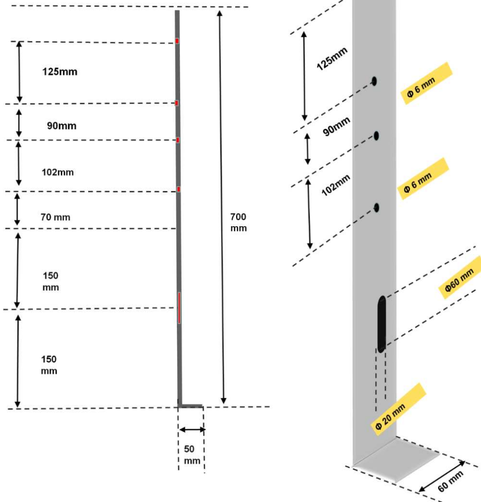
Εικόνα 17. Σχέδιο γωνιακού μεταλλικού ελάσματος για ταυτόχρονη τοποθέτηση ανακλαστήρων WWR και οπτικοακουστικών απωθητών πάνω στο μεταλλικό στηθαίο του αυτοκινητόδρομου.
